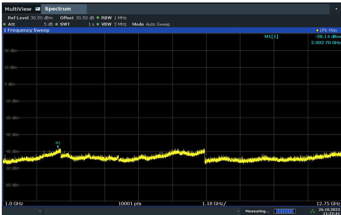
图4-9 1GHz~12.75GHz 频段
