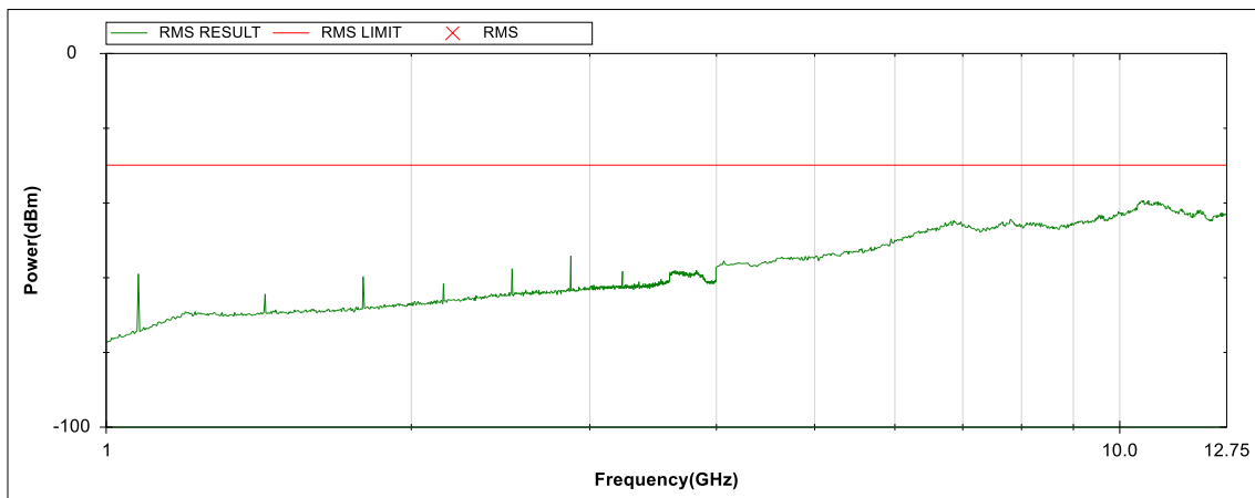
图4-11 1GHz~12.75GHz 频段
