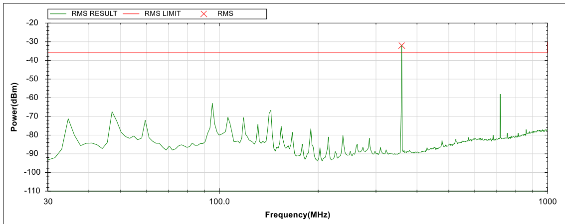
图4-10 30MHz~1GHz 频段
